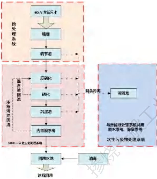
图 7.2-1 项目生活污水处理工艺流程图
