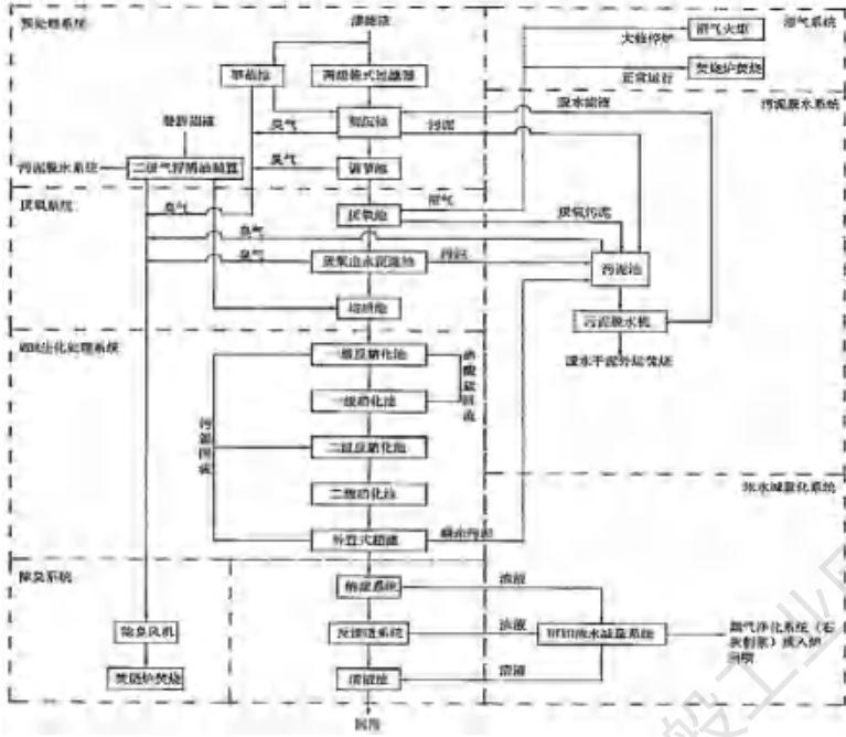
图 3.3-4 渗滤液处理工艺流程图
