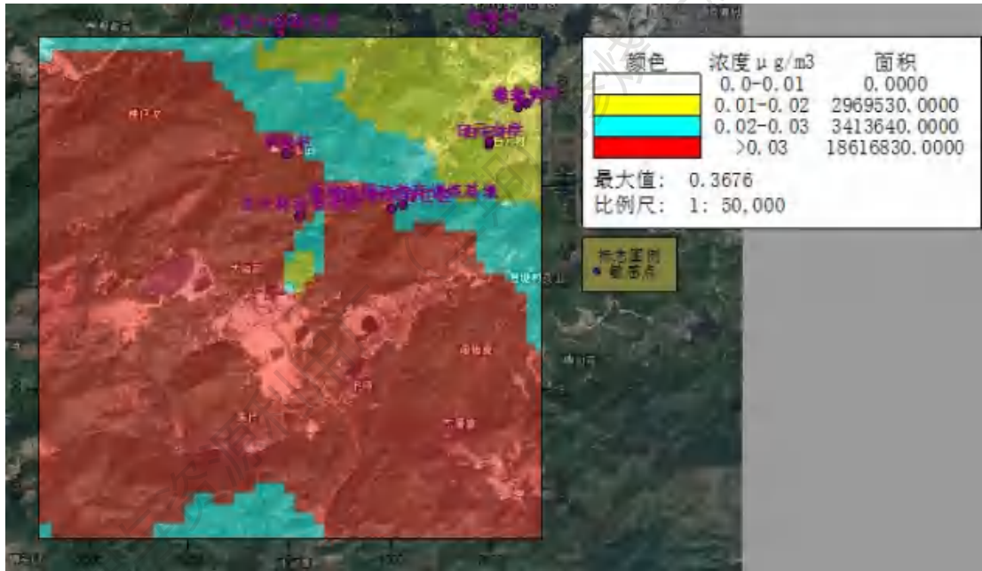
图6.2-12 \text{PM}_{10} 年平均浓度贡献值图
