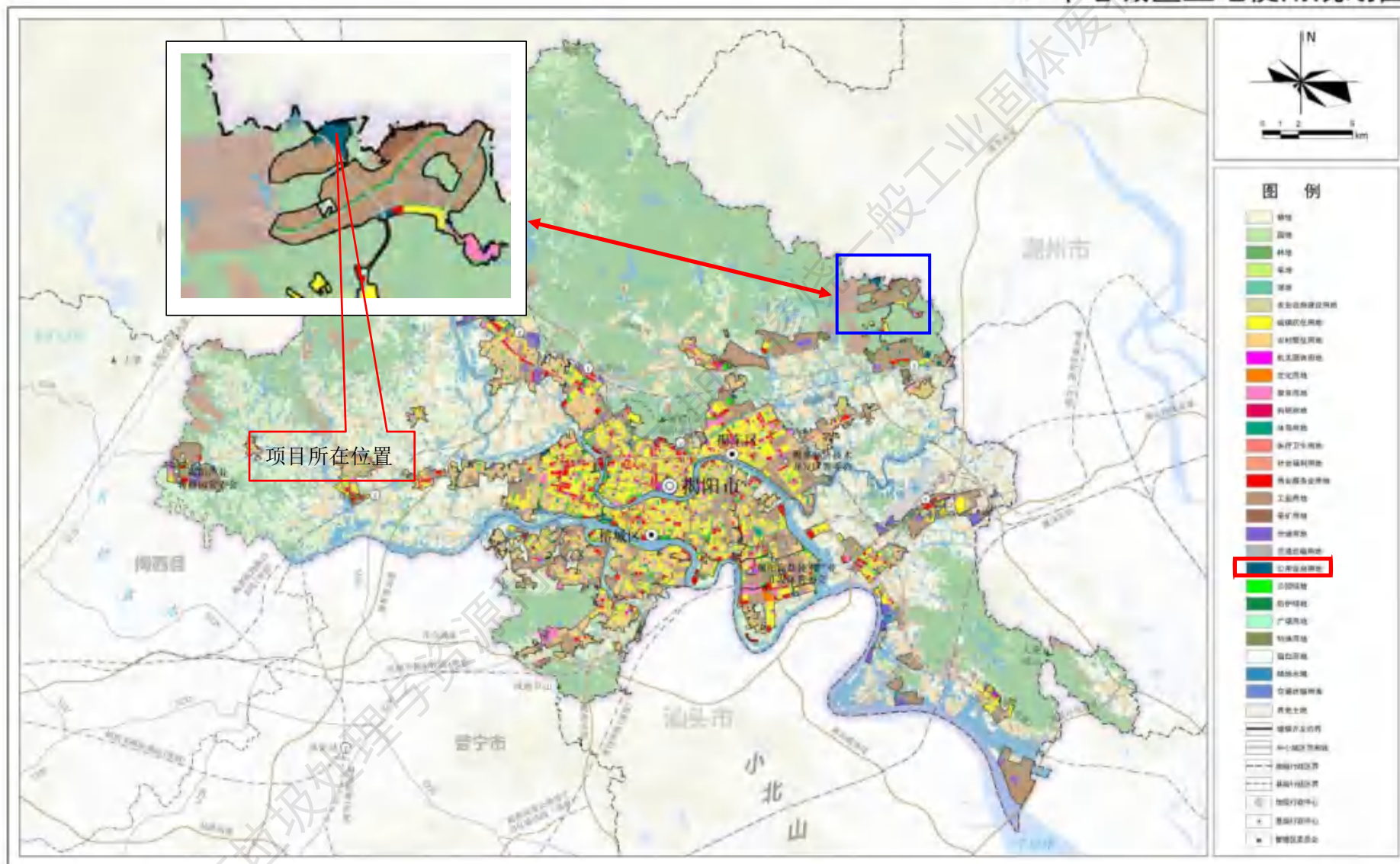
36 中心城区土地使用规划图
