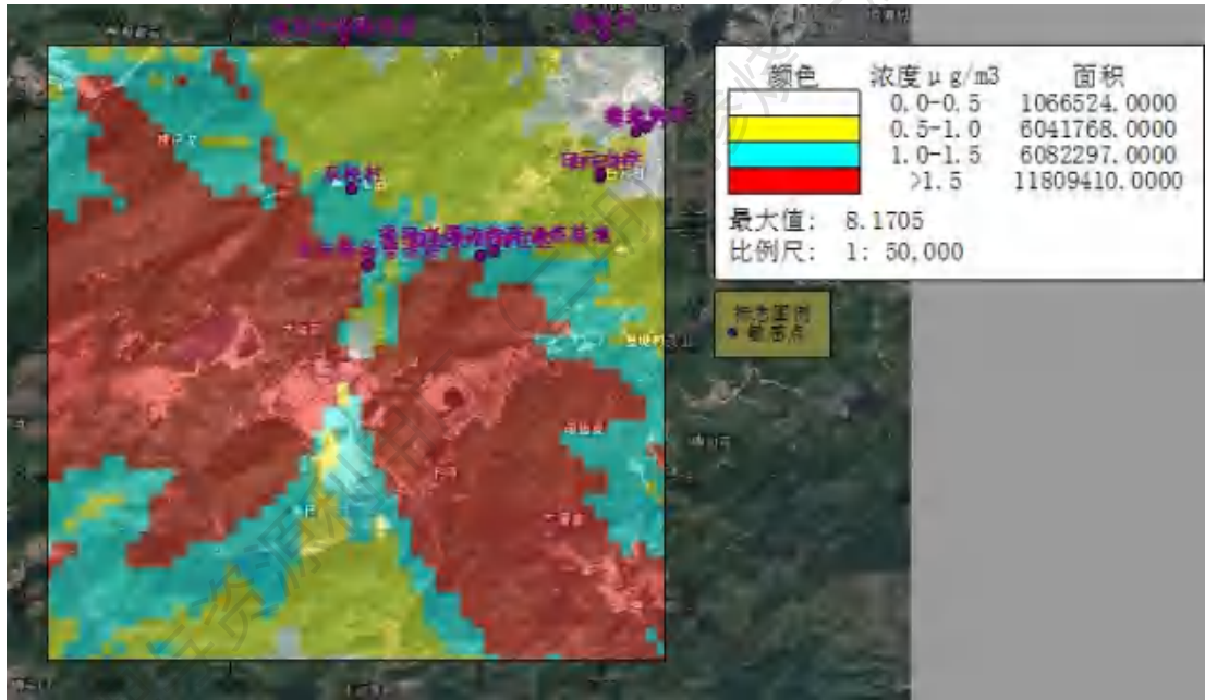
图6.2-16 CO 日平均浓度贡献值图
