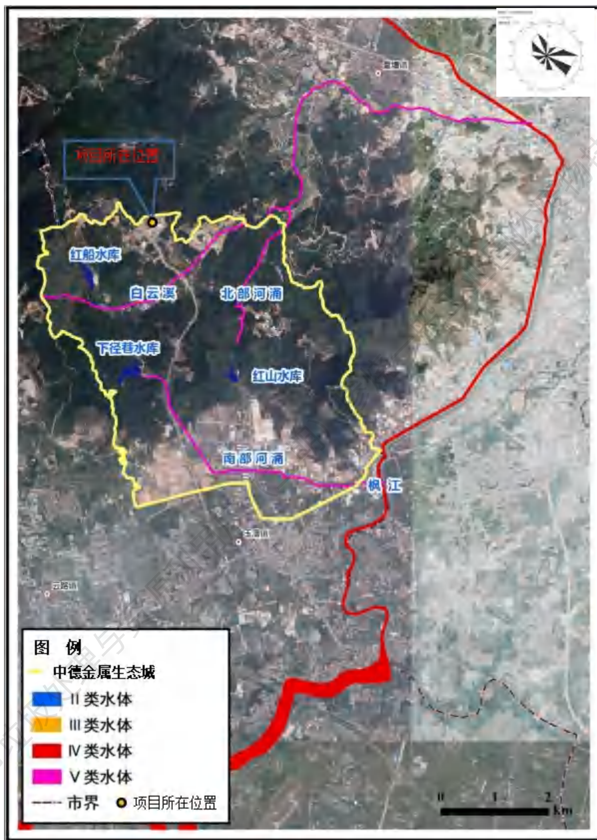
图 2.2-4 本项目项目所在周边水系图
