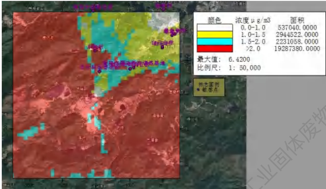
图6.2-17 HCl 1小时平均浓度贡献值图
