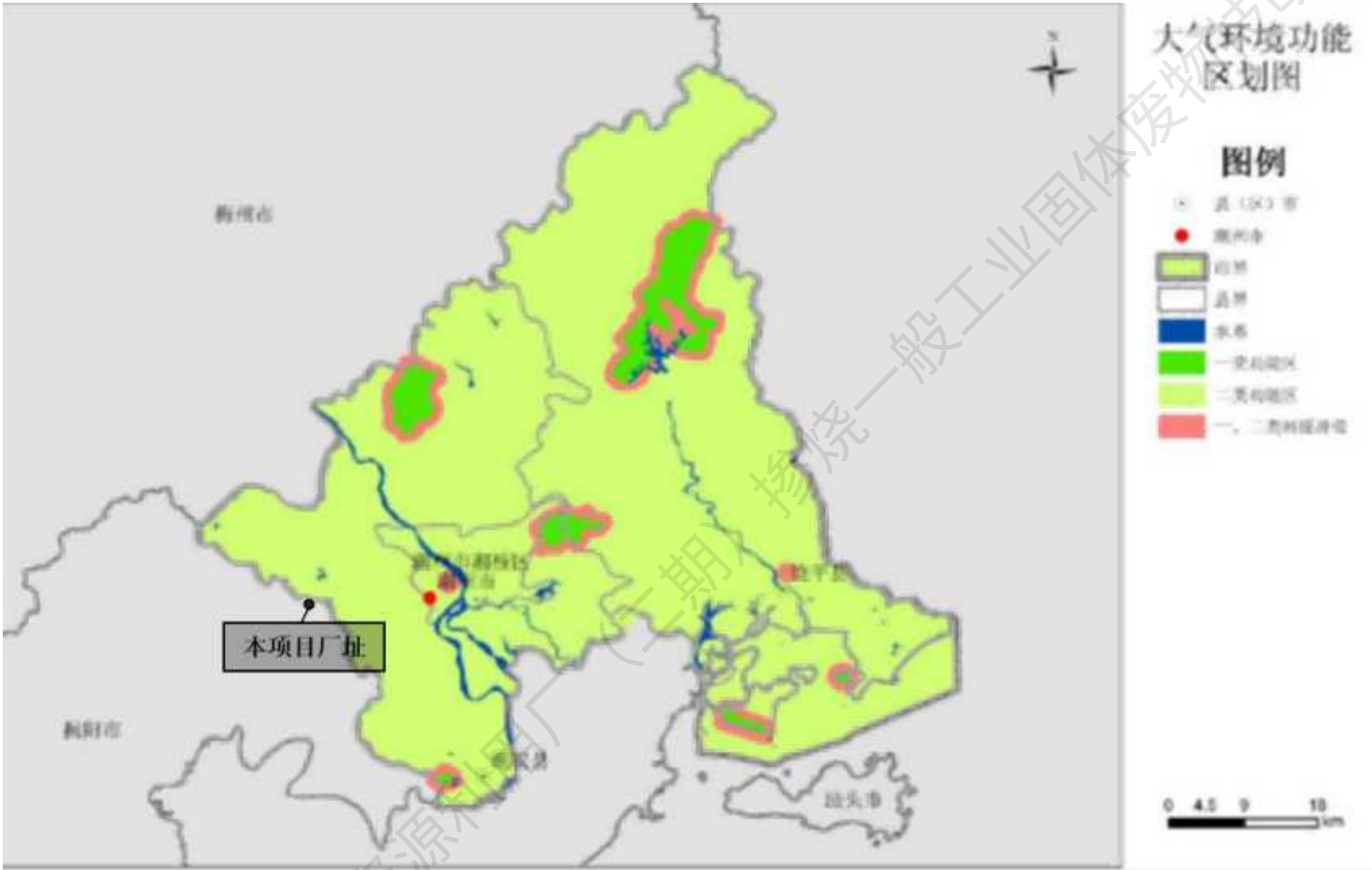
图 2.2-2 项目临近的潮州市域内的大气环境功能区划图
