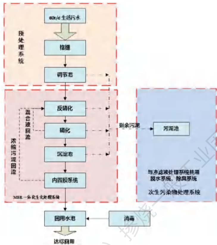
图 3.3-2 生活污水处理工艺流程图
