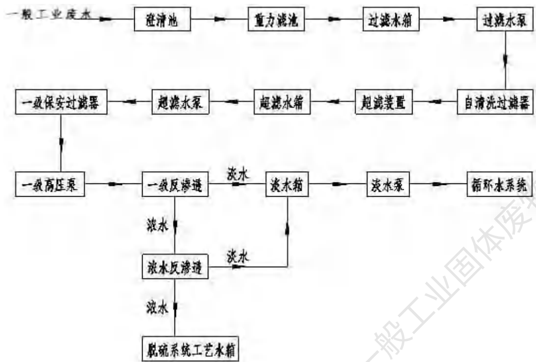
图 7.2-2 项目工业废水处理工艺流程图
