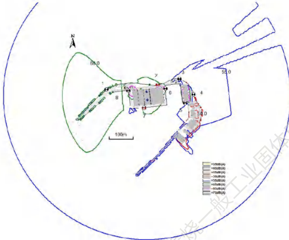
图 6.4-2 非正常工况下噪声预测等声值线图
