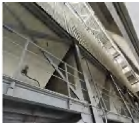
焚烧炉烟气处理-布袋除尘器
