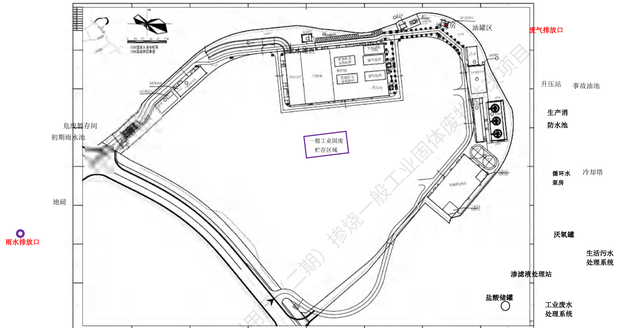
图 4.1-1 技改项目平面布置图（依托原有项目）
