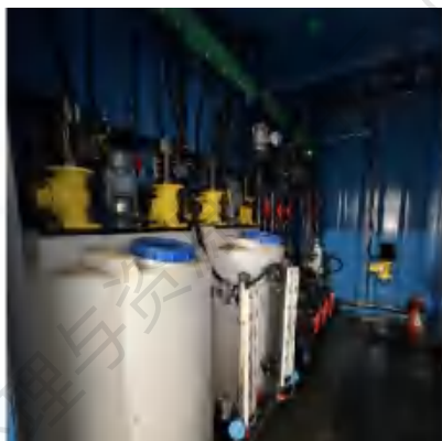
生活污水处理（MBR一体化生化系统）
