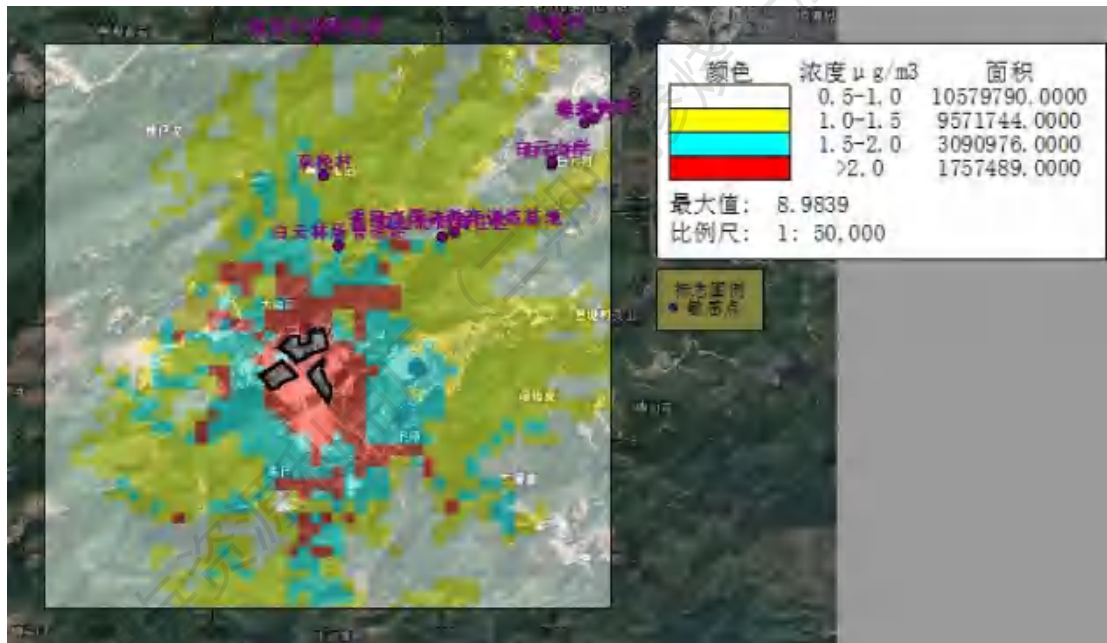
图6.2-36 \text{H}_2\text{S} 1小时平均浓度预测值图
