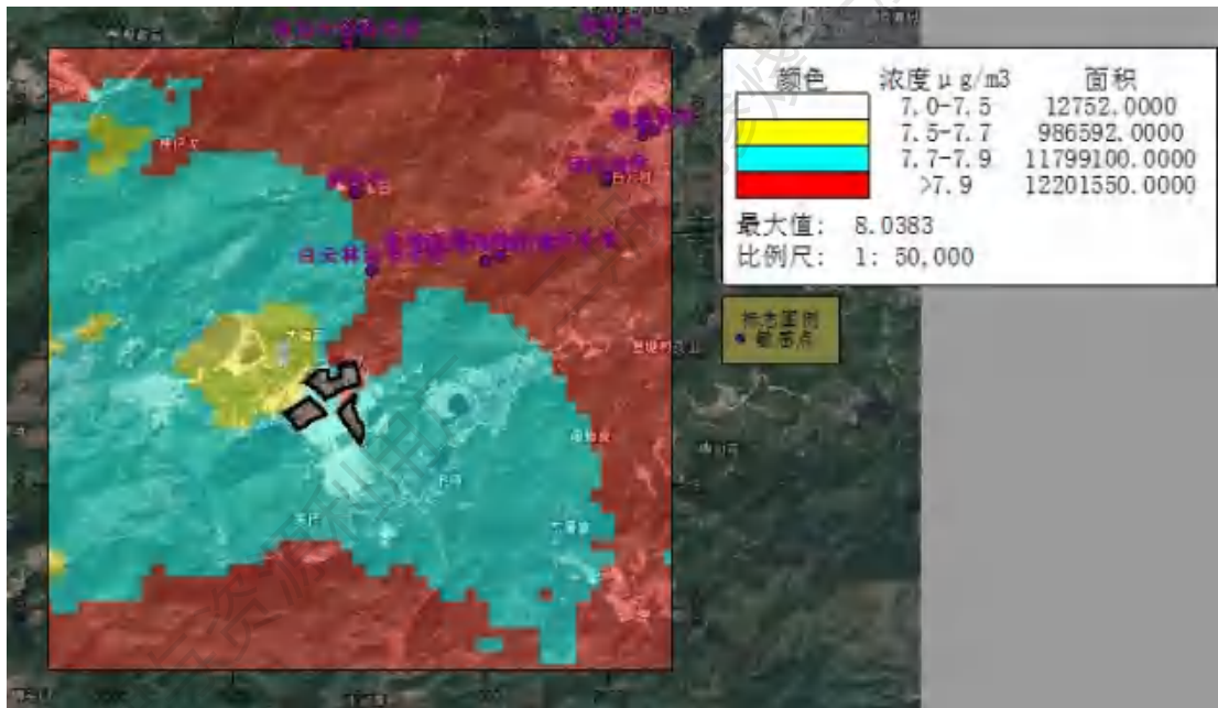
图6.2-26 \text{SO}_2 年平均浓度预测值图
