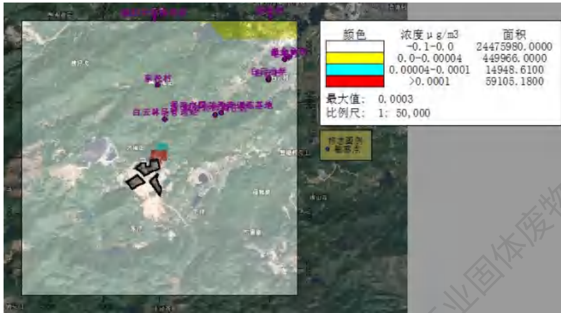
图6.2-39 Pb 年平均浓度预测值图
