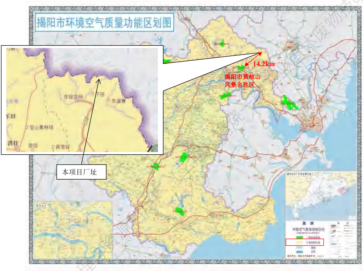
图 2.2-1 项目所在地的大气环境功能区划图
