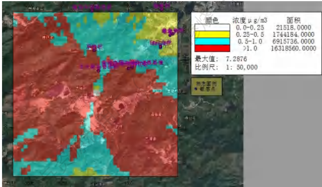
图6.2-6 SO 2 日平均浓度贡献值图
