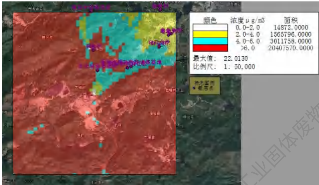
图6.2-5 SO 2 1小时平均浓度贡献值图
