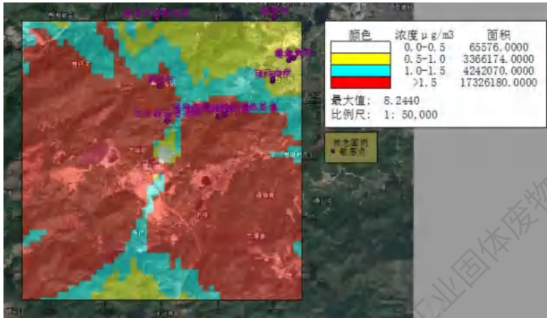
图6.2-9 NO 2 日平均浓度贡献值图
