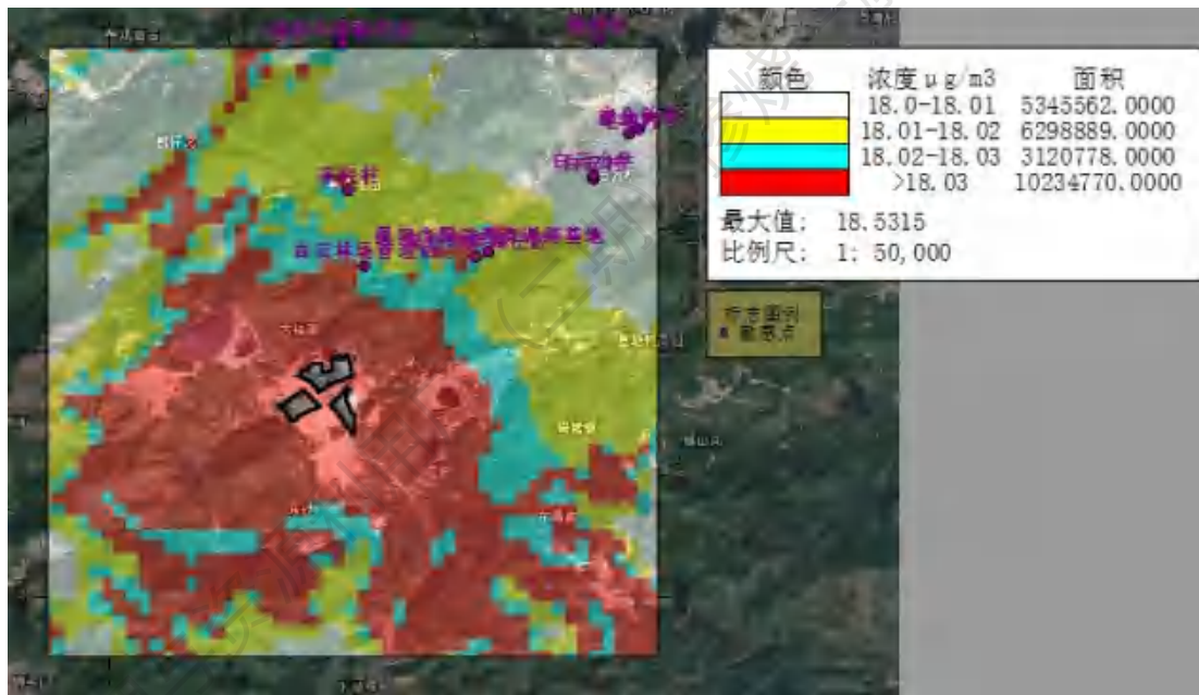
图6.2-28 \text{NO}_2 年平均浓度预测值图
