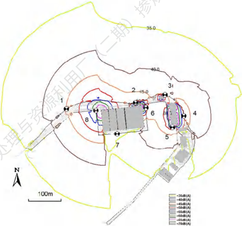
图 6.4-1 正常工况下噪声预测等声值线图
