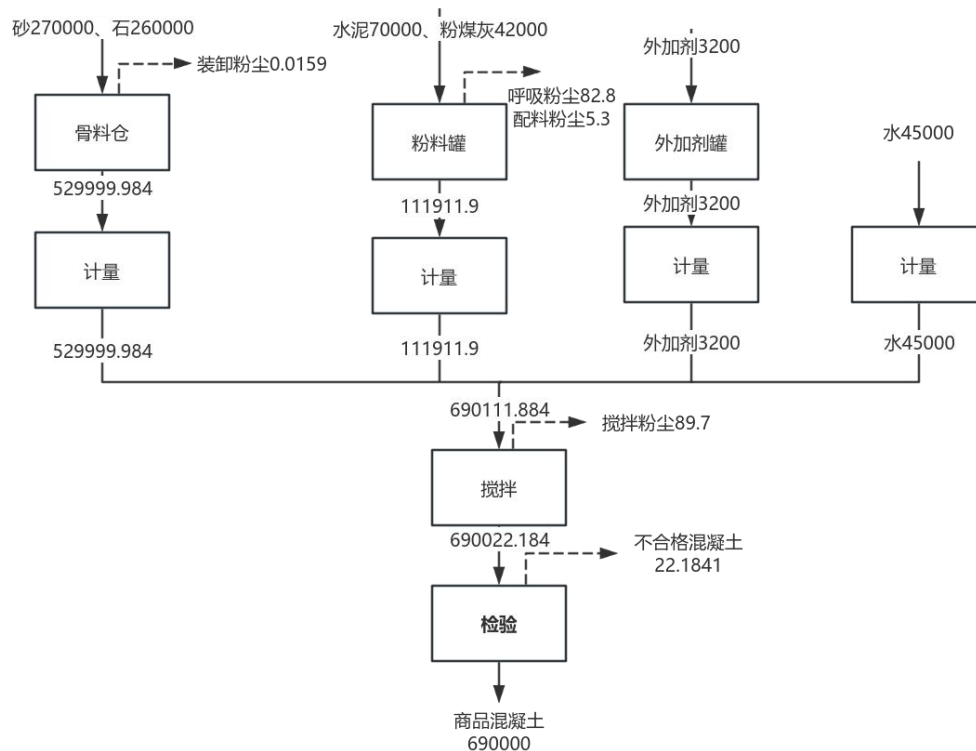
图 2-2 项目物料平衡图 (t/a)
