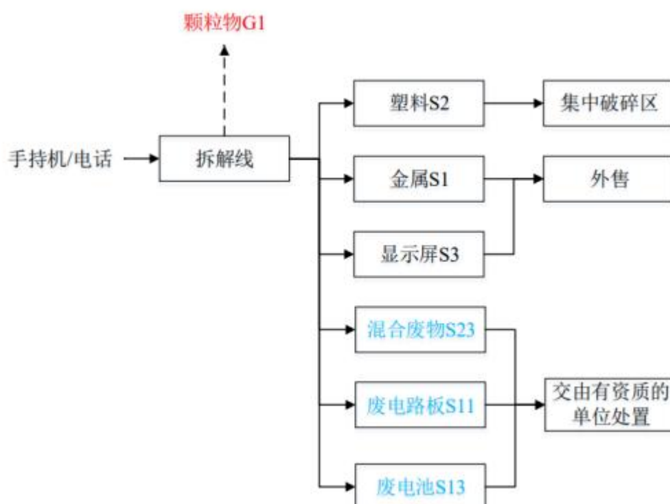
图 2-8 废移动通信手持机/电话单机拆解工艺流程图
