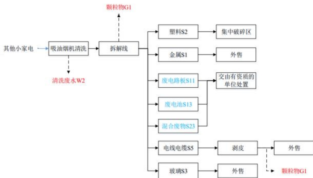
图 2-10 其他小家电拆解工艺流程图
