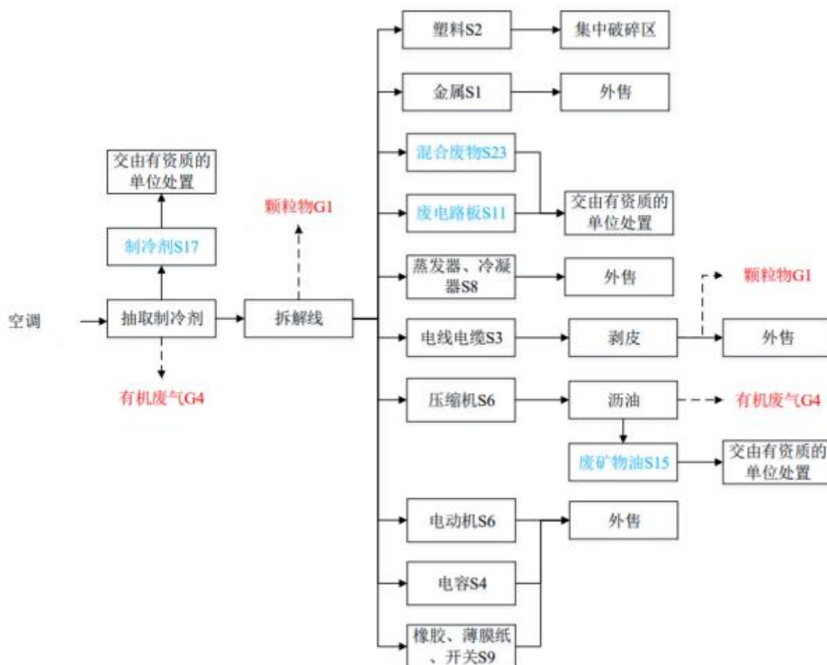
图 2-6 空调器拆解工艺流程图
