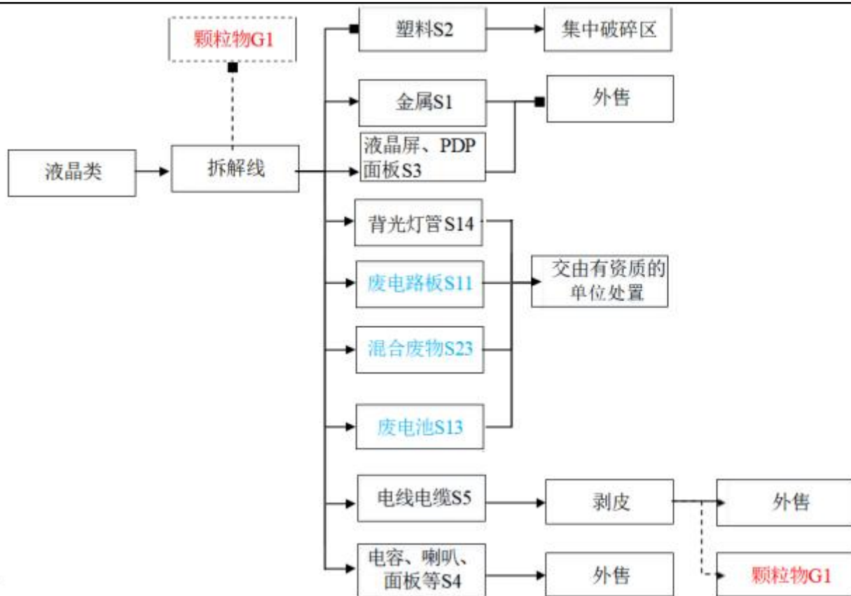
图 2-4 废液晶类电视机、电脑显示器及监视器拆解工艺流程图
