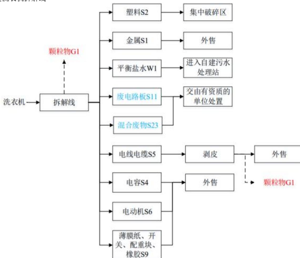
图 2-7 废洗衣机拆解工艺流程图
