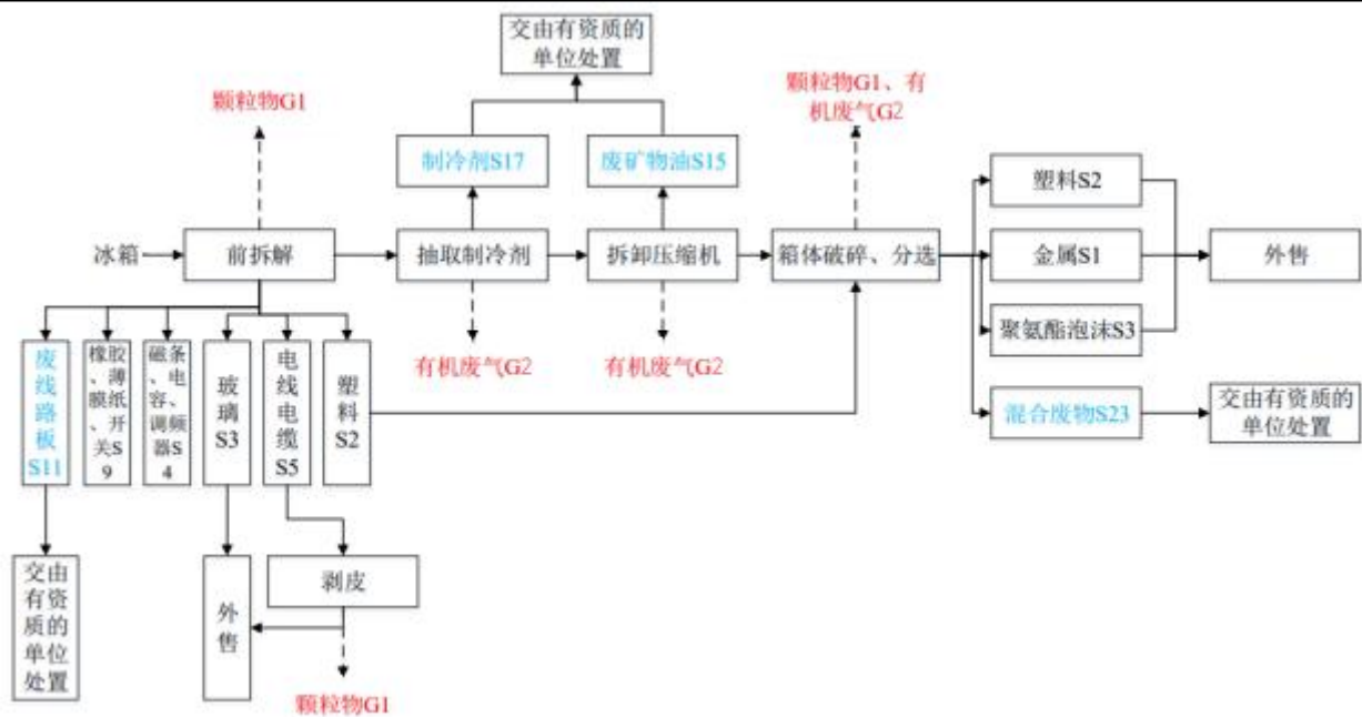
图 2-5 废电冰箱拆解工艺流程图
