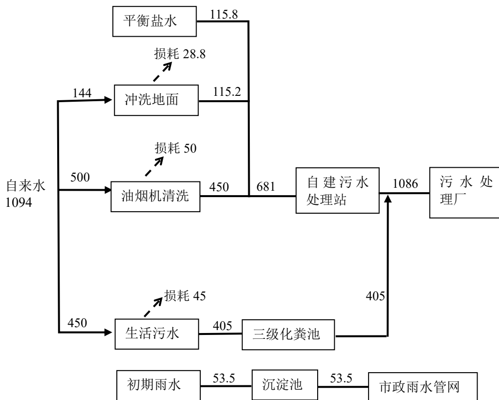
图 4-1 项目水平衡图 (m³/a)
