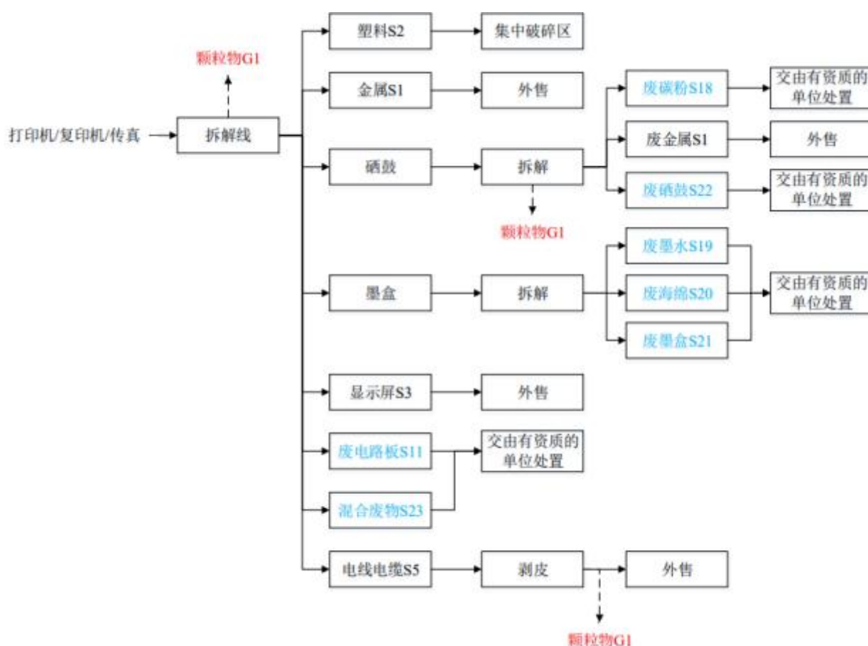
图 2-9 废打印机/复印机/传真机拆解工艺流程图
