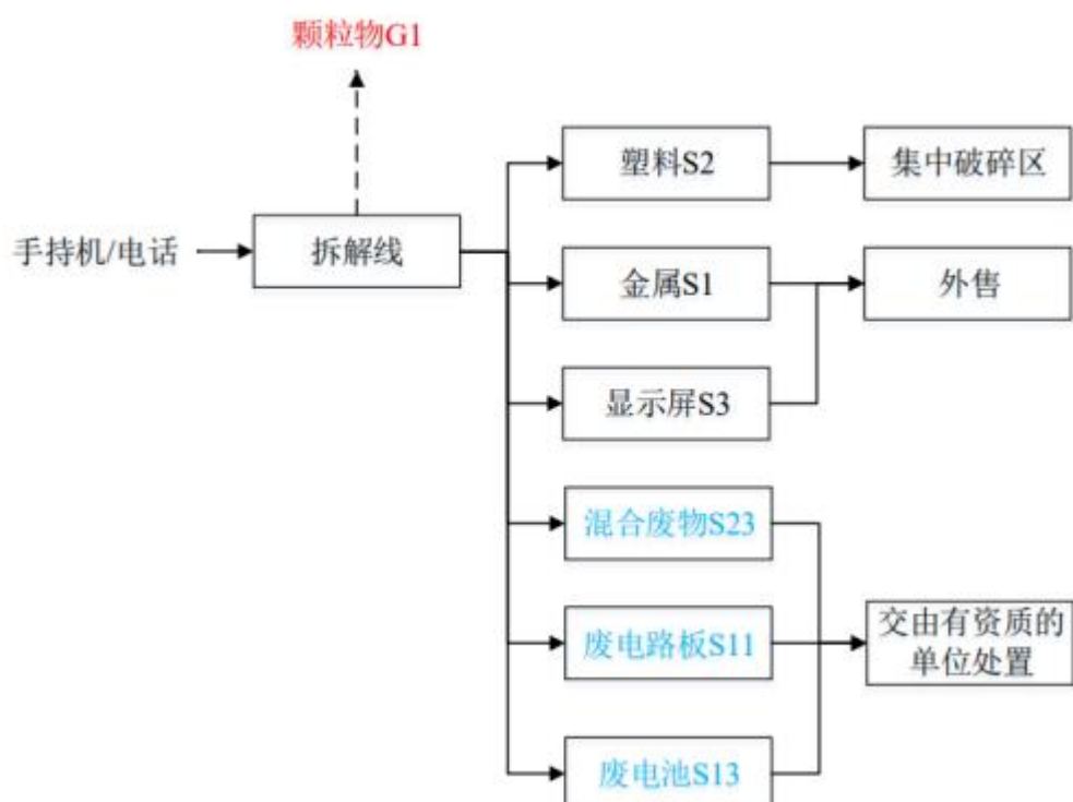
图 2-5 废移动通信手持机/电话单机拆解工艺流程图
