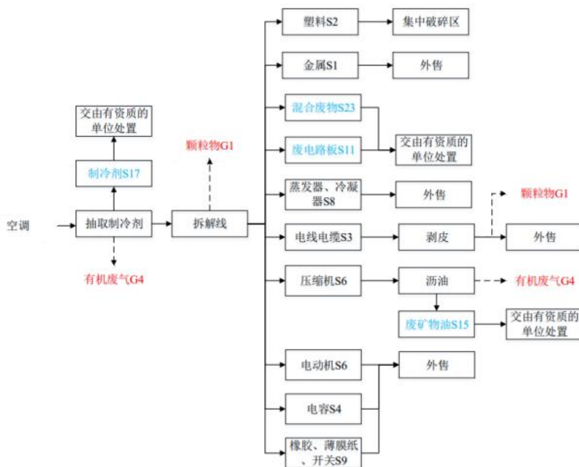
图 2-3 废空调器拆解工艺流程图
