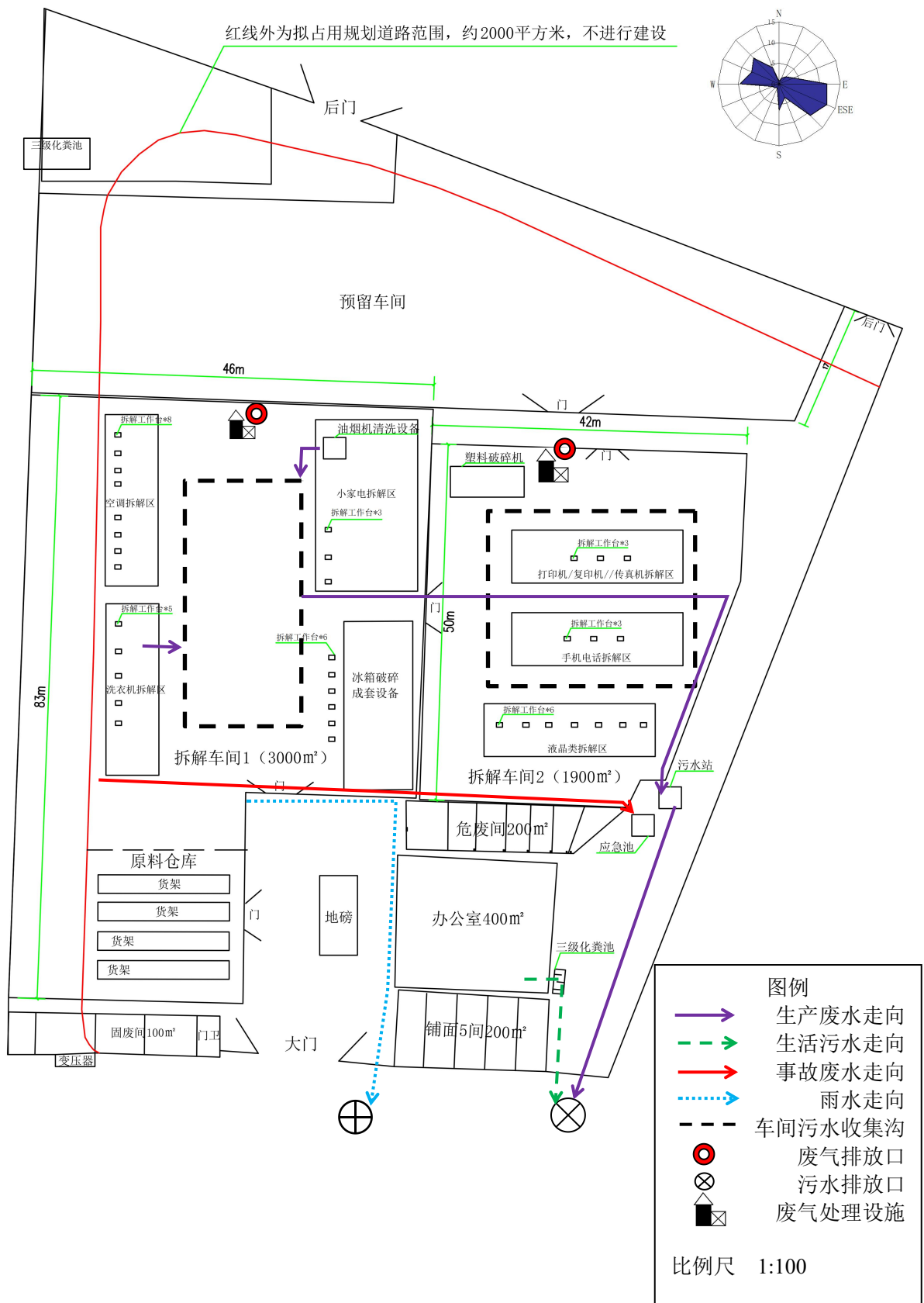
附图 4 项目总平面图
