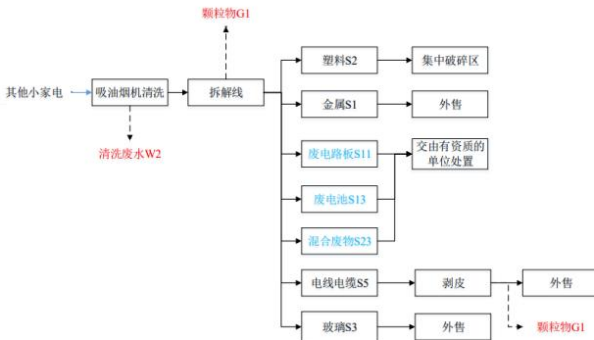
图 2-7 其他小家电拆解工艺流程图
