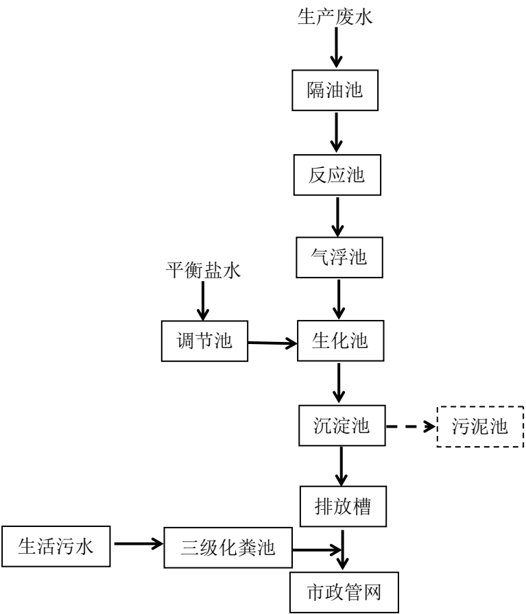
图 4-2 项目废水处理工艺流程图
