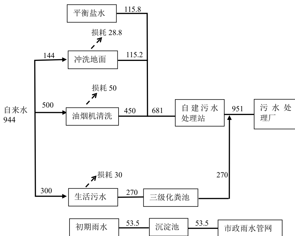
图 4-1 项目水平衡图 (m³/a)
