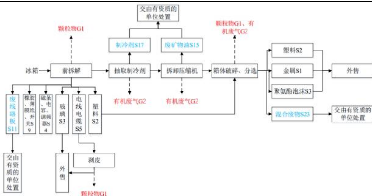
图 2-2 废电冰箱拆解工艺流程图
