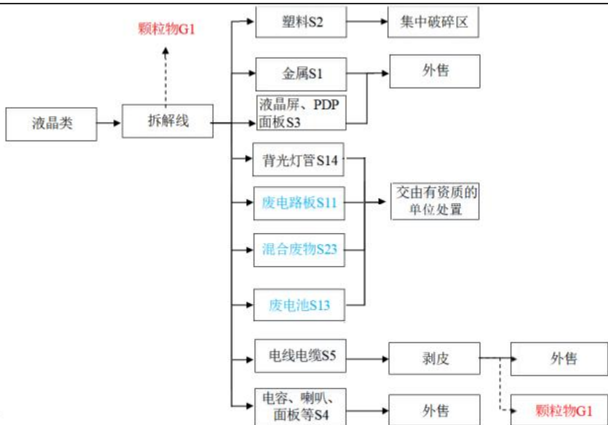
图 2-1 废液晶类电视机、电脑显示器及监视器拆解工艺流程图
