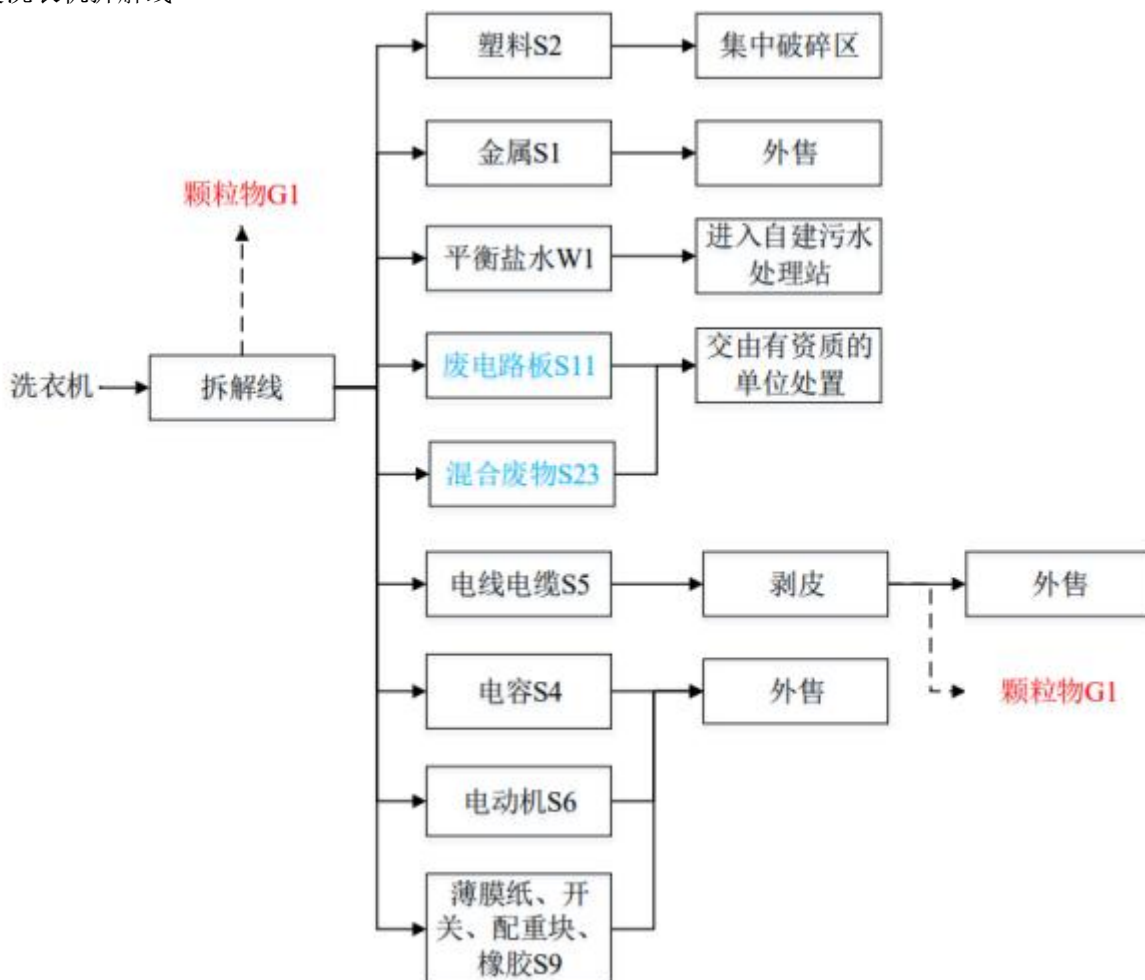
图 2-4 废洗衣机拆解工艺流程图
