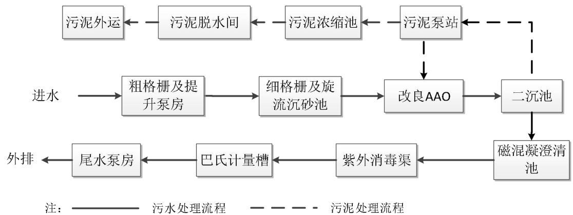
图 4-3 揭阳市榕城区北部水质净化厂工艺流程图
