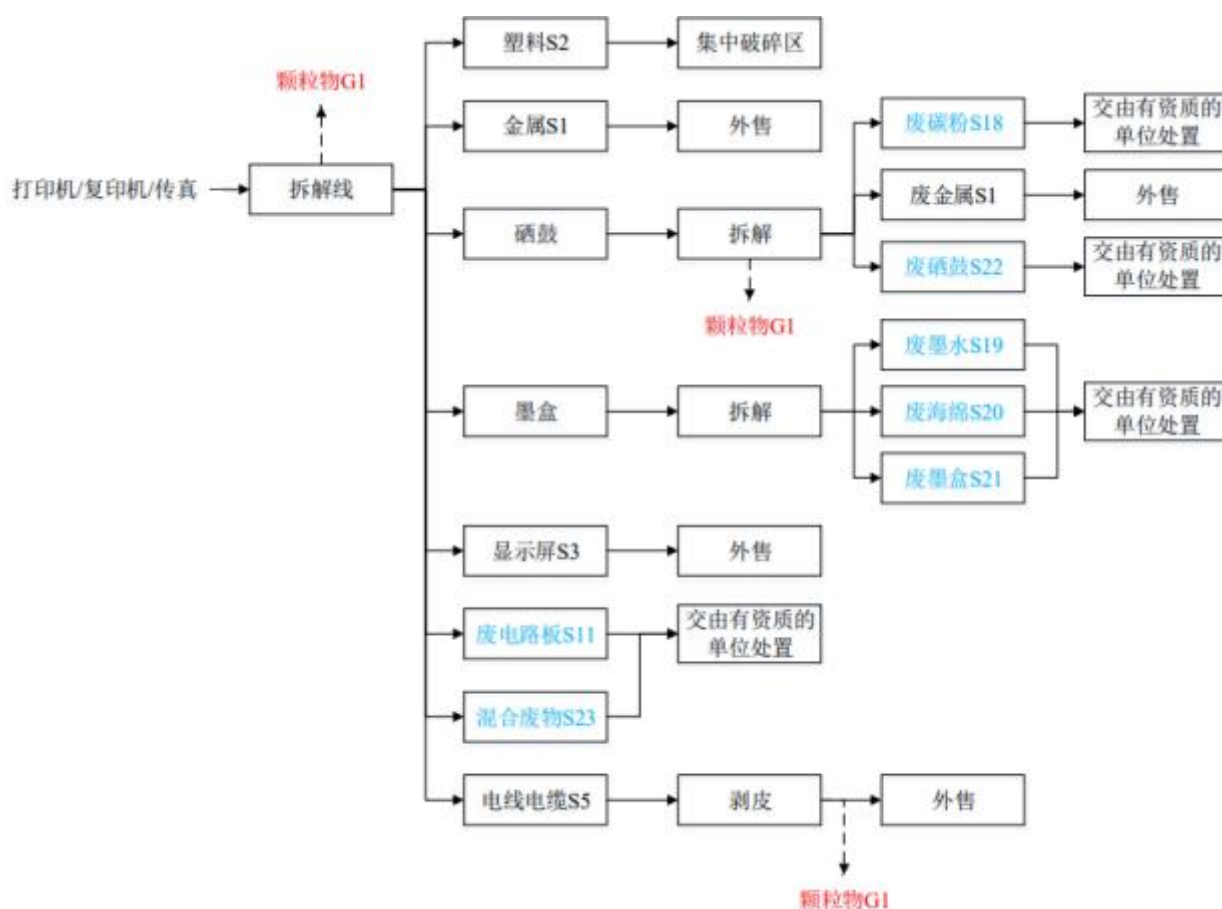
图 2-6 废打印机/复印机/传真机拆解工艺流程图
